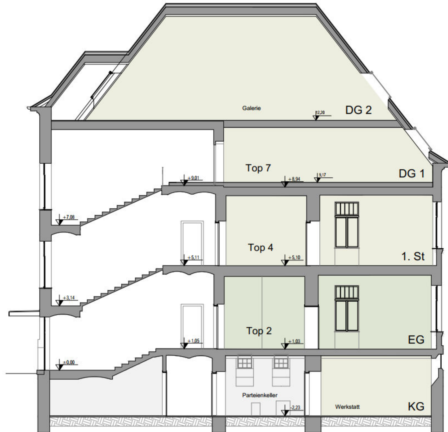
Schnitt A-A
